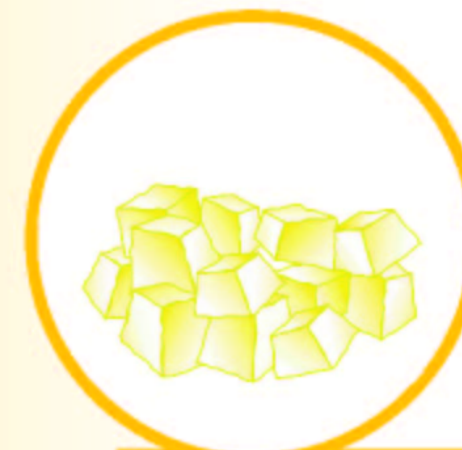
Сера
